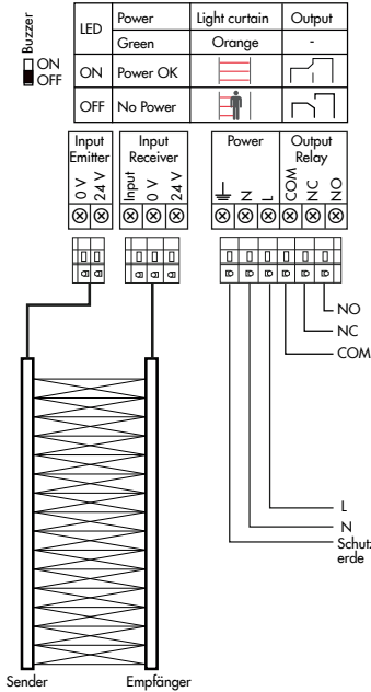
Abb 9: Verkabelung des UPS mit einem Lichtvorhang
