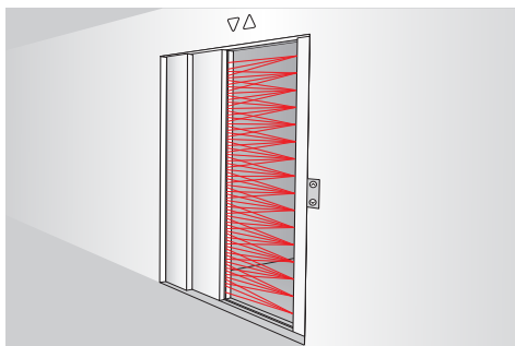
Figur 2: Statisk applikation
