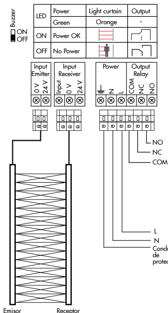
Figura 9: Cableado de la UPS con una barrera fotoeléctrica
