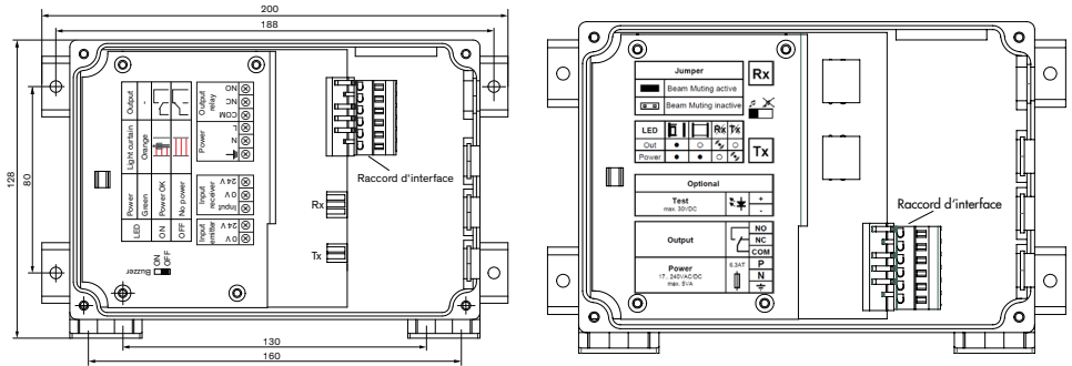
Figure 4: L'alimentation UPS possède le même raccord d'interface de l'entraînement de porte que la commande cegard/Max et dispose donc d'une compatibilité descendante.
