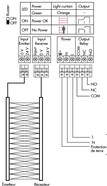
Figure 9: Câblage de l'alimentation UPS avec un rideau lumineux
